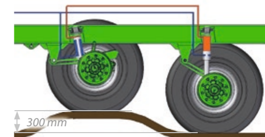
Wszystkie modele ROYAL są wyposażone w wysokiej jakości agregat 4-resorowy . Zapewnia on wysoką sztywność konstrukcyjną, komfort jazdy i sprawność.
