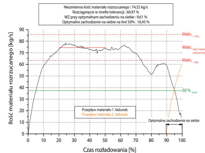
Adapter rozrzucający 2-Spread z dwoma pionowymi walcami.
